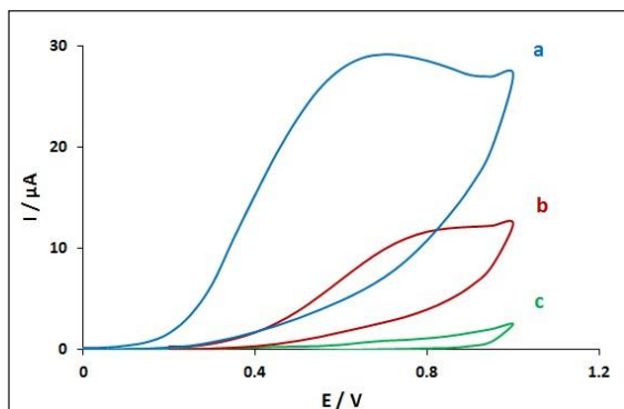
شکل ۲ ولتاموگرام‌های چرخه‌ای هیدرازین (با غلظت ۱/۰ میلی‌مولار در محلول بافر فسفات ۰/۱ مولار با \text{pH}=8 ) در سطح الکترواد خمیر کربن اصلاح‌شده با نانوذرات استرانسیم فریت نمودار (a)؛ در سطح الکترواد خمیر کربن اصلاح‌نشده نمودار (b)؛ نمودار (c) پاسخ الکترواد اصلاح‌شده در محلول بافر را نشان می‌دهد.
