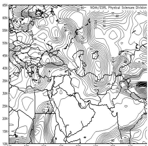
شکل ۱۰- نقشه رطوبت نسبی در روز ۲۲ مهر ماه ۱۳۹۱
