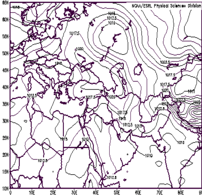
شکل ۷- نقشه تراز سطح دریا در روز ۲۲ مهر ماه ۱۳۹۱ (روز
