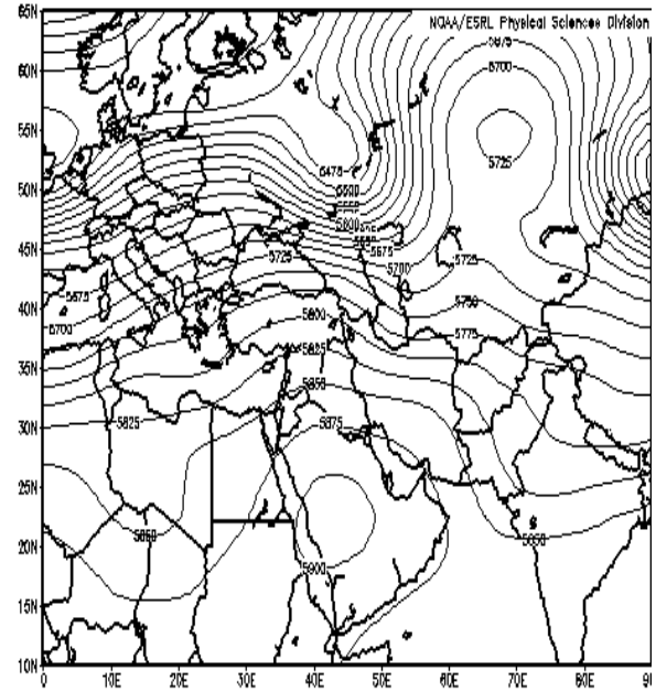
شکل ۸- نقشه تراز ۵۰۰ هکتوپاسکال در روز ۲۲ مهر ماه
