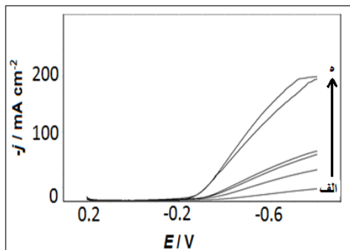
شکل ۷ ولتاگرام‌های روبش خطی فرایند آزادسازی هیدروژن در سطح Pt-CNT/CPE در سولفوریک اسید با غلظت‌های (الف) 0.1، (ب) 0.3، (ج) 0.05، (د) 0.075، (ی) 0.1 و (ه) 0.2M با سرعت روبش 100 mV s⁻¹
