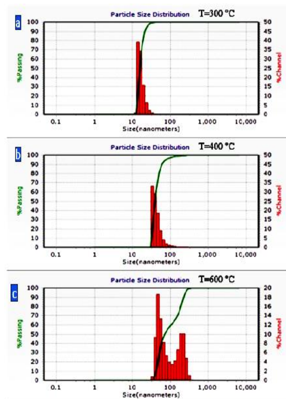
شکل ۵: نمودار DLS، دمای کوره (a) ۳۰۰، (b) ۴۰۰ و (c) ۶۰۰°C.
