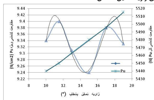
شکل ۵. اثر زاویه تمایل بشقاب گاوآهن بشقابی بر مقاومت کششی کل و ویژه
