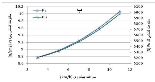
شکل ۴. اثر سرعت پیشروی بر مقاومت کششی کل و ویژه گاوآهن
