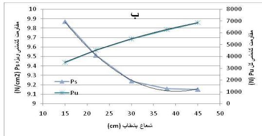
شکل ۳. مقاومت کل و ویژه گاوآهن‌های برگرداندار (الف) و بشقابی
