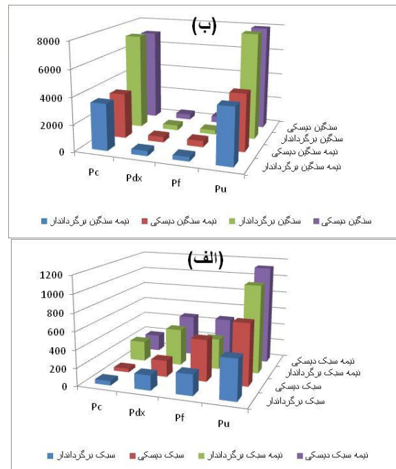
شکل ۱. الف) اثر خاک دارای بافت سبک و نیمه سبک و ب) نیمه سنگین و سنگین بر مقدار مقاومت ناشی از برش خاک ( P_c )، مقاومت ناشی از جابجایی خاک ( P_{dx} )، مقاومت ناشی از اصطکاک خاک با فلز ( P_f ) و مقاومت کل عامل خاک‌ورز ( P_u ) گاوآهن‌های برگرداندار و بشقابی
