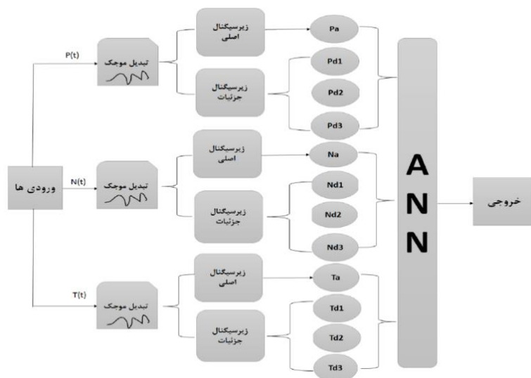
شکل ۳: نمای شماتیکی از مدل موجک- شبکه عصبی
